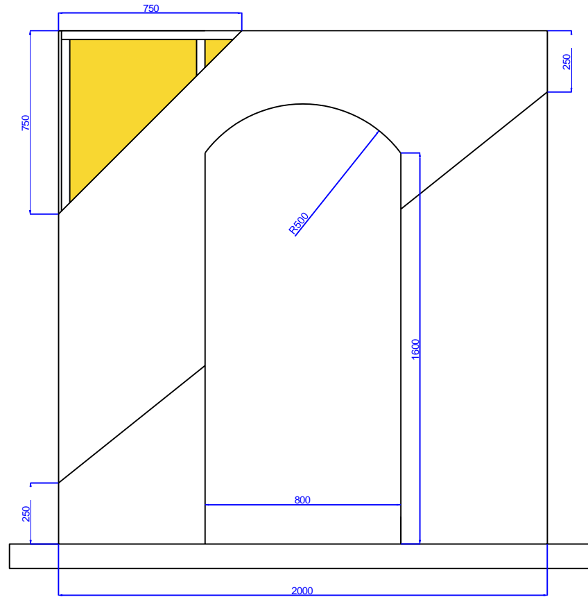
ELEVATION B
