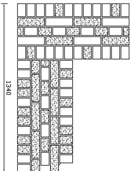
Elevation B
