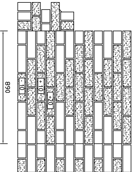
Elevation A
