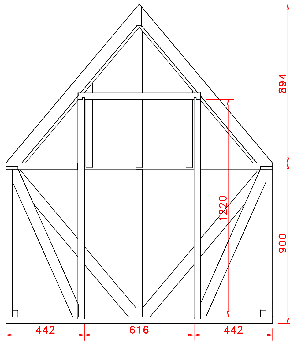
ELEVATION
