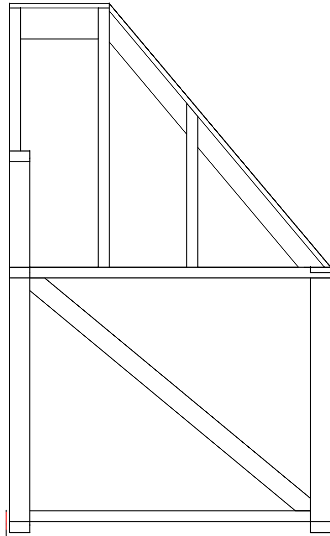
END ELEVATION
