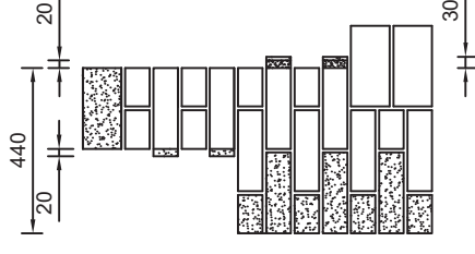
End Elevation
